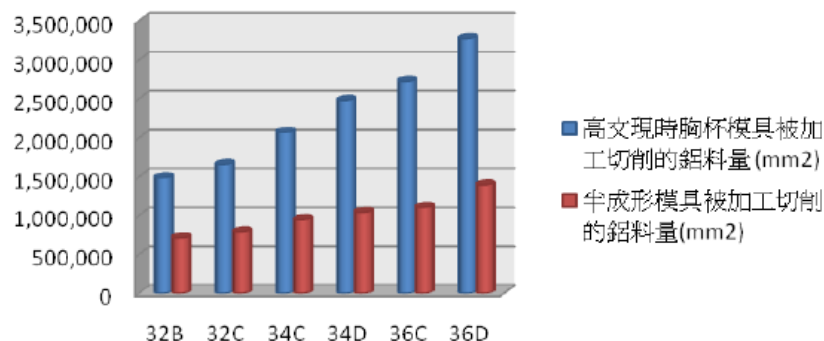
胸杯模具加工被切削的鋁料
